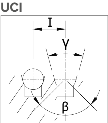
Gargantas en U con subranura
