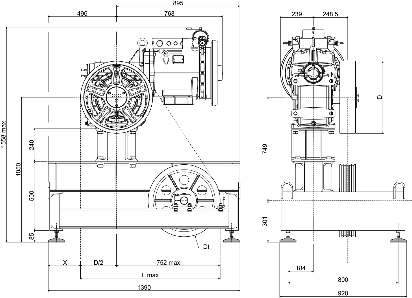
XTE5708 (Dt 400-450-520) (silentblocks incluidos) Peso de las bancadas: 293 kg. (bancadas + polea de desvío + silentblocks)
