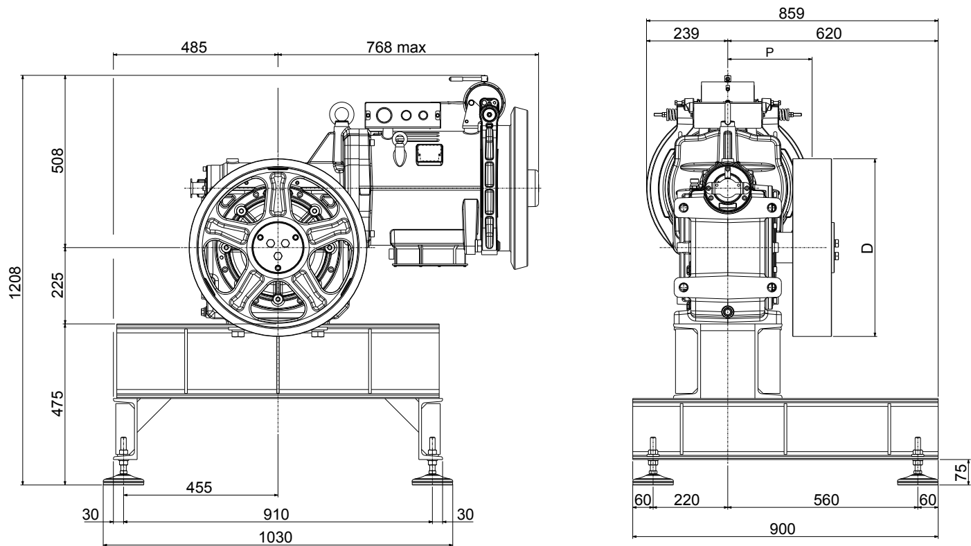
XTE5706 (D 450-700) (silentblocks incluidos) Peso de las bancadas: 108 kg (bancadas + silentblocks)
