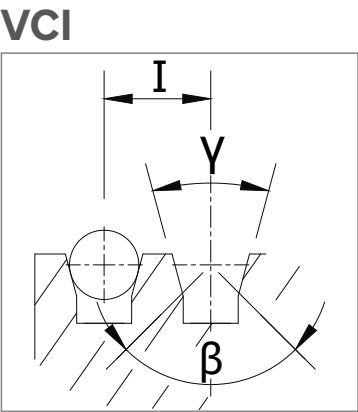
Gargantas en V con subranura
