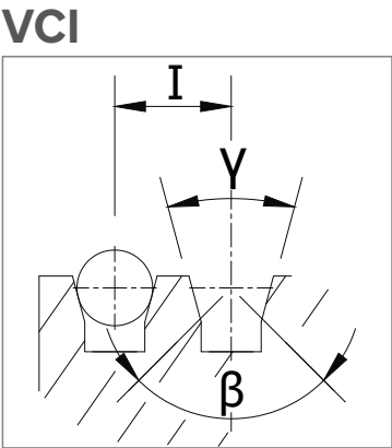
Gargantas en V con subranura
