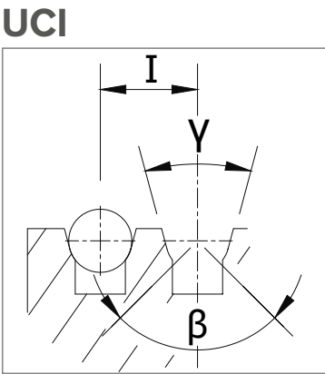
Gargantas en U con subranura
