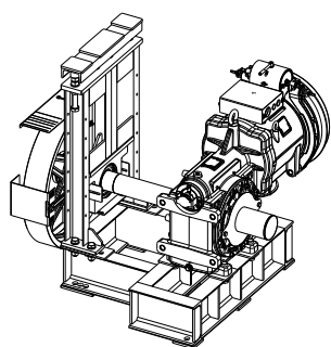
Máquina derecha
